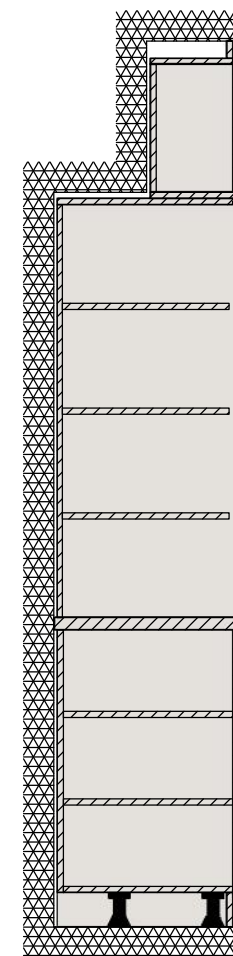
ŘEZ D - D
